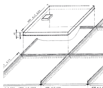
MINIMÁLNÍ VZDÁLENOSTI *
